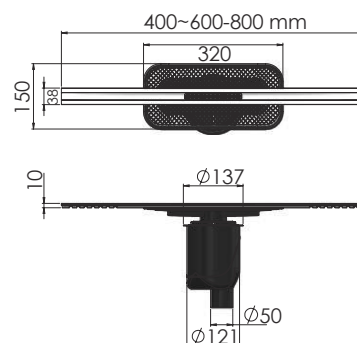
Вертикальный S-образный сифон D50/105мм - H30/80мм - 48L/min
