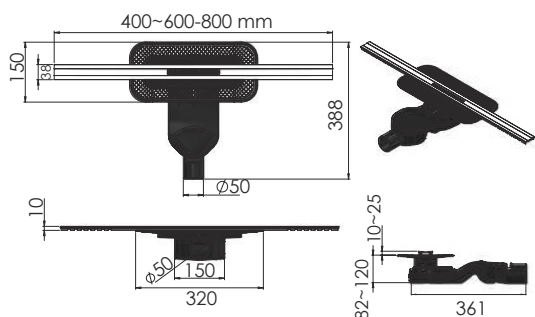
Боковой S-образный сифон D50-H80-60L/min
