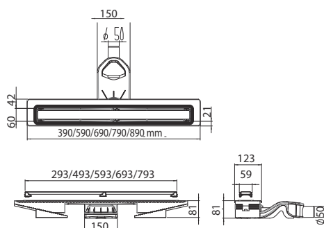
Боковой S-образный сифон D50-H80-60L/min
